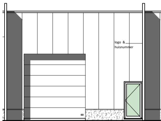
Elekt. sectionaal poort 4000 br x 4200 h
