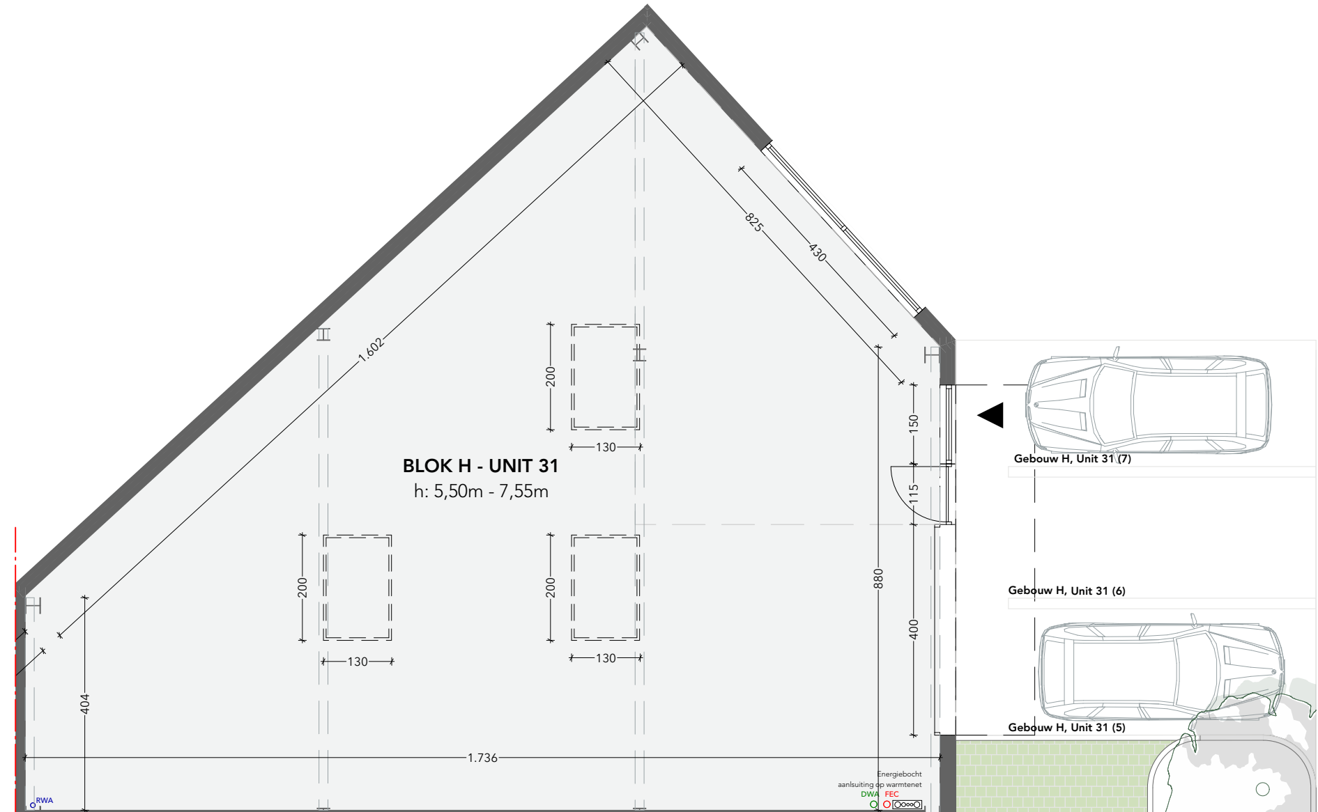
Grondplan
