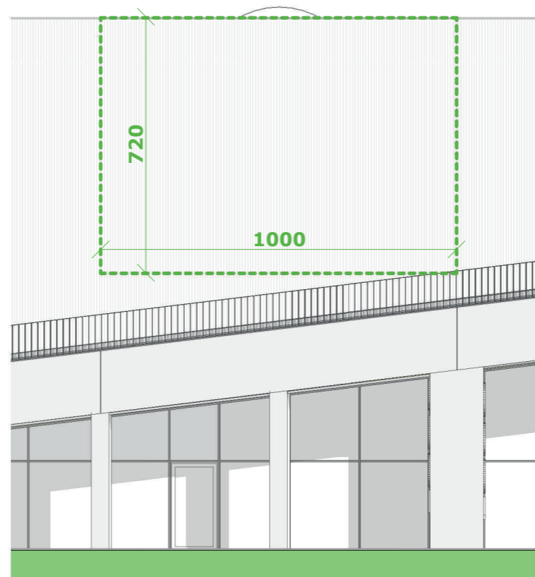
Zuidgevel
