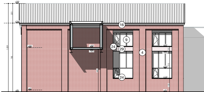
Zijgevel
