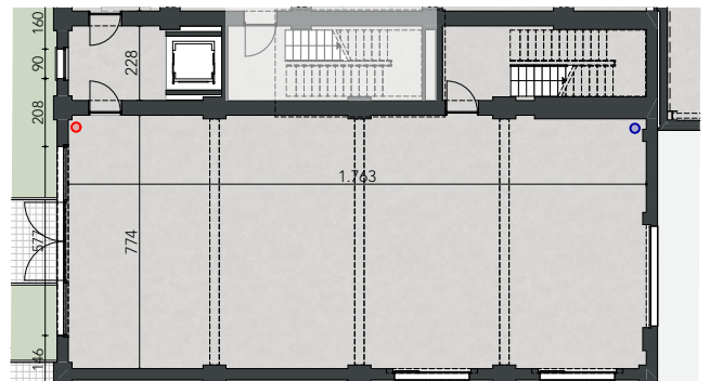
Gelijkvloers
