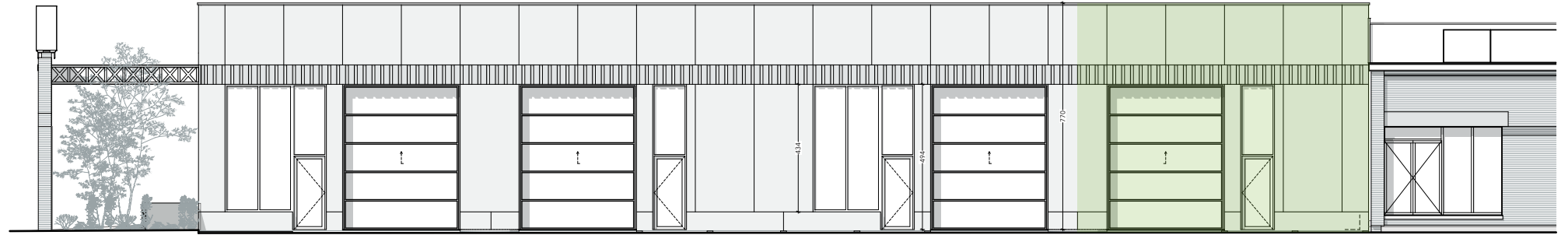
Voorgevel
